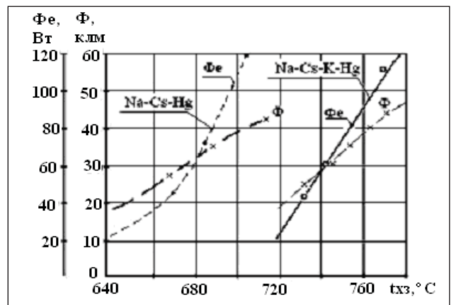
Рис. 4. Залежність потоку випромінювання (Фе) і світлового потоків ( \Phi ) випромінювання натрієвих ламп потужністю 400 Вт із добавками цезію та калію від температури холодної зони t_{xz}
