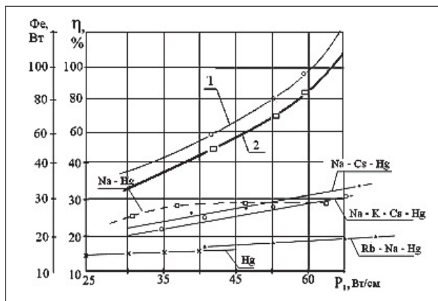
Рис. 3. Залежність енергетичного потоку випромінювання (Фе) з різними добавками (1-Cs(5%); 2-K(1%), Cs(5%)) та світлової ефективності ( \eta ) ламп із різним наповненням (□ – Na-Hg, о – Na-K-Cs-Hg, • – Na-Cs-Hg, × – Hg, ▲ – Rb-Na-Hg) від питомої потужності ламп ( P_1 )
